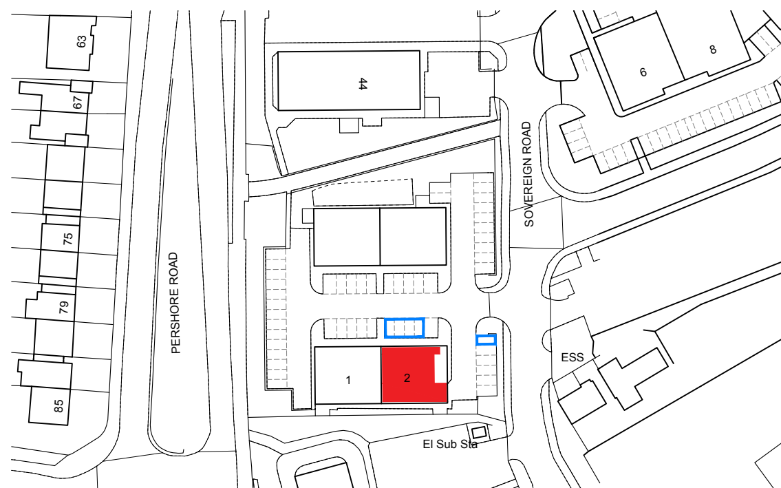
Site Plan 1.1250
